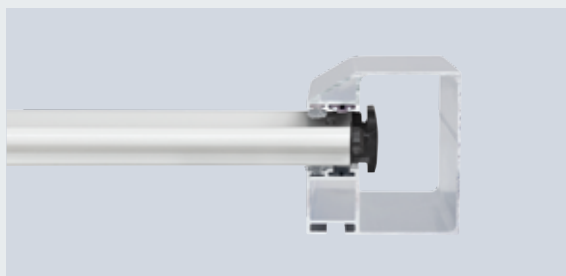
Rolovací vrata DD s profilem Decotherm S a plastovým větrným hákem
